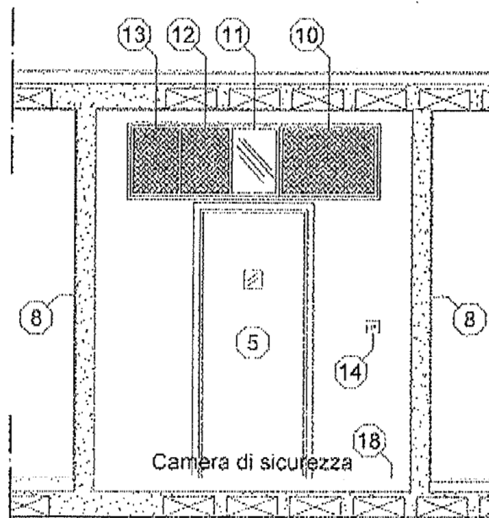
Sezione B-B
