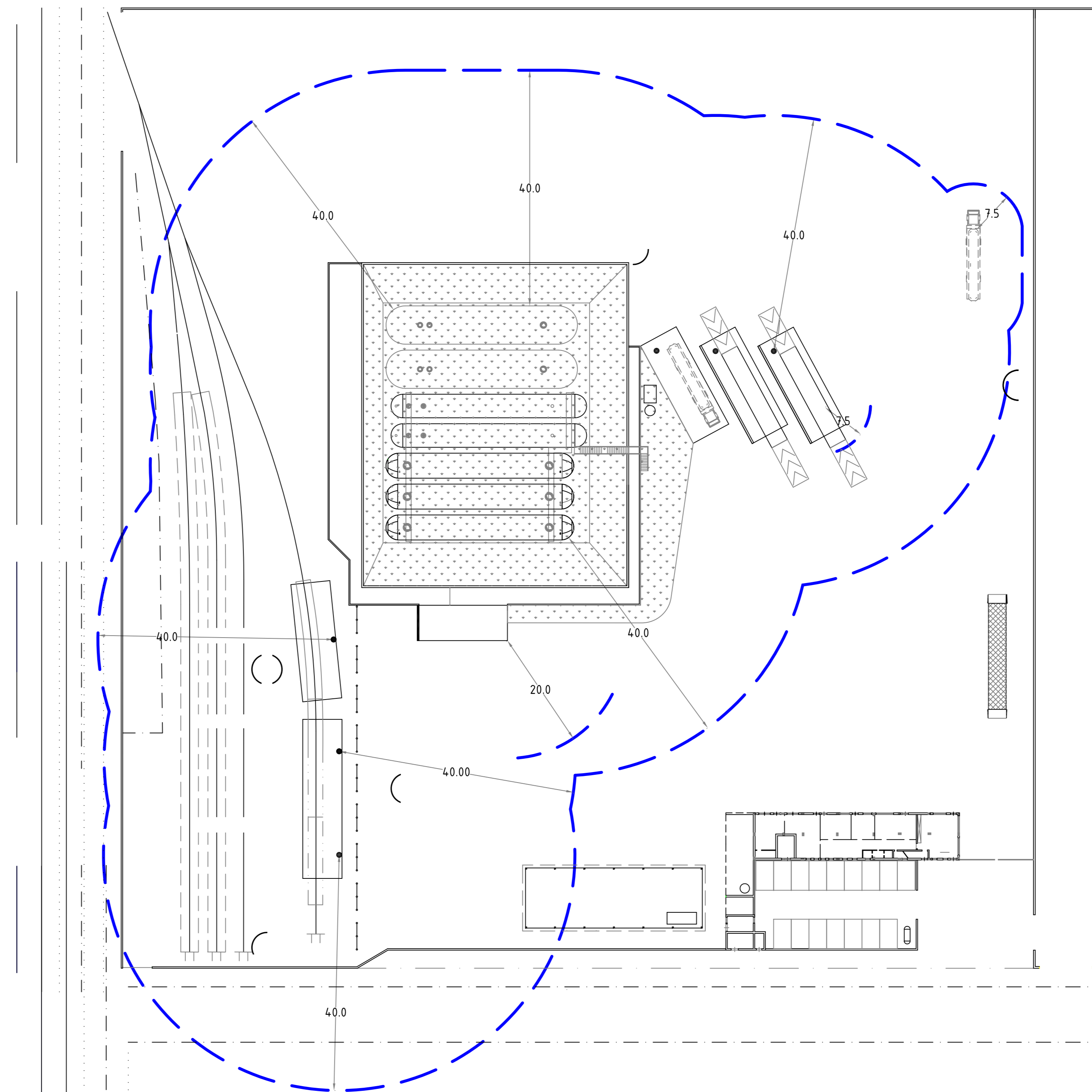
Distanze di sicurezza esterne (scala 1:500)
