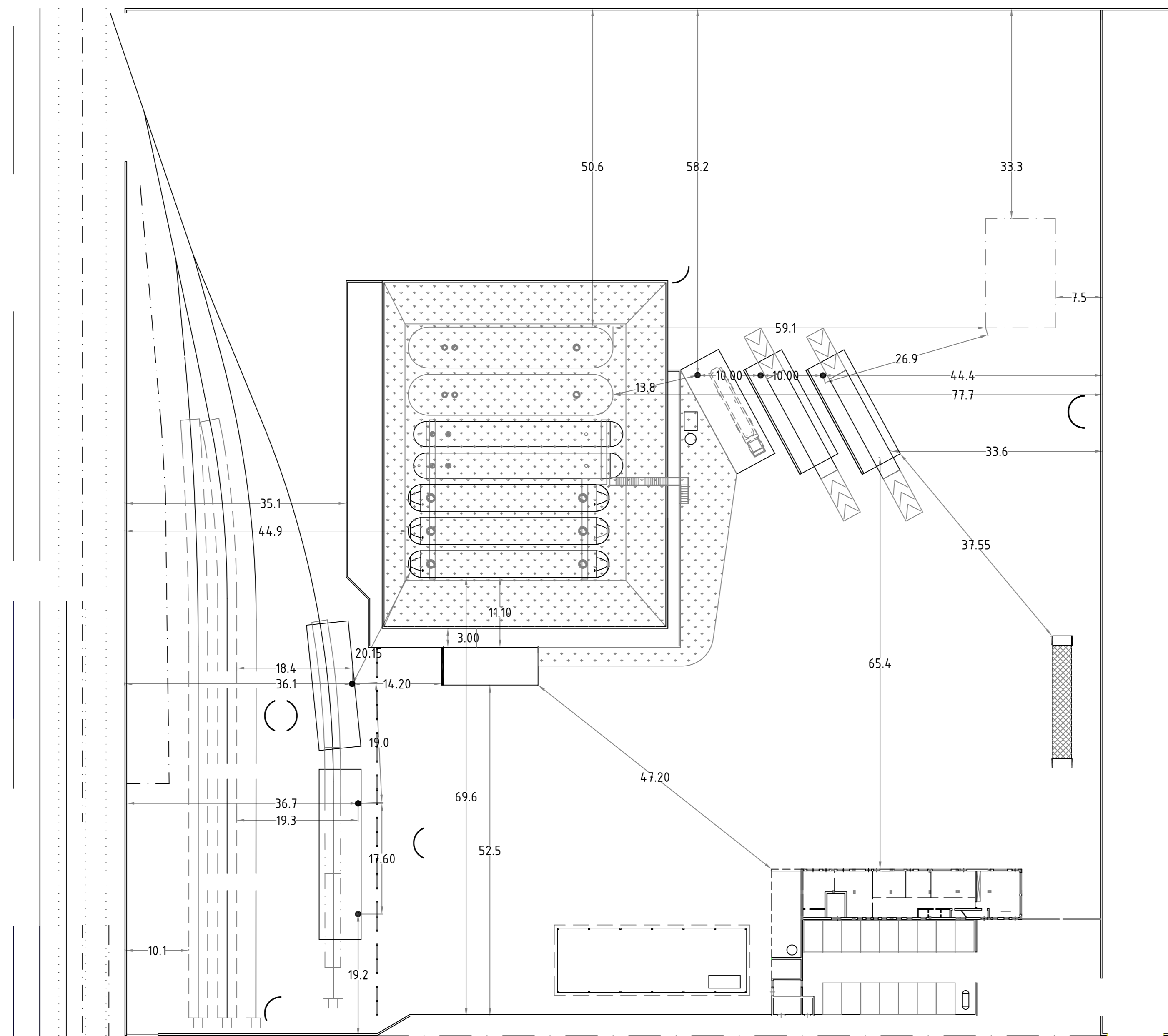
Distanze di sicurezza interne e di protezione (scala 1:500)
