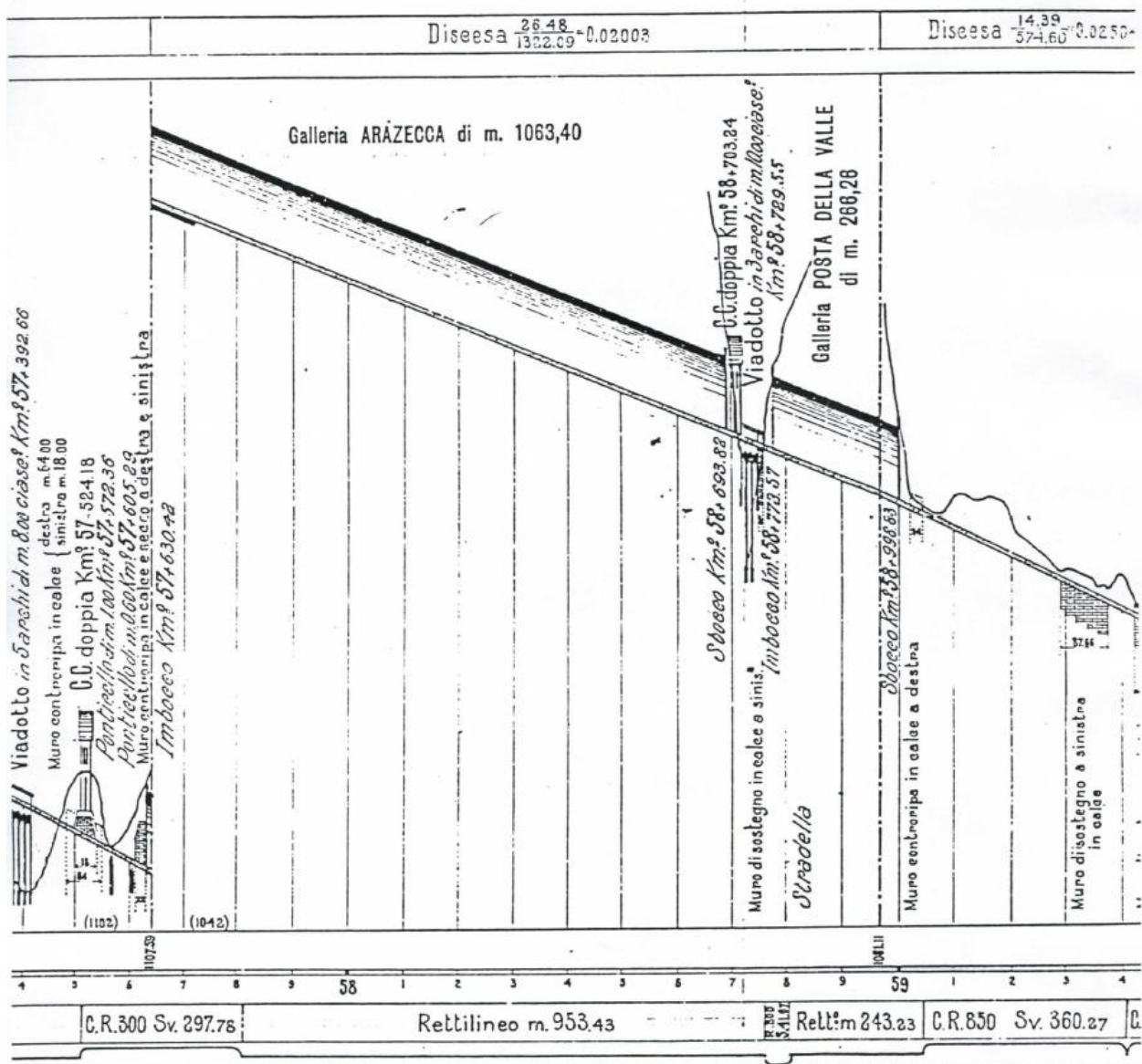
Stralcio del profilo plano-altimetrico della linea ferroviaria
