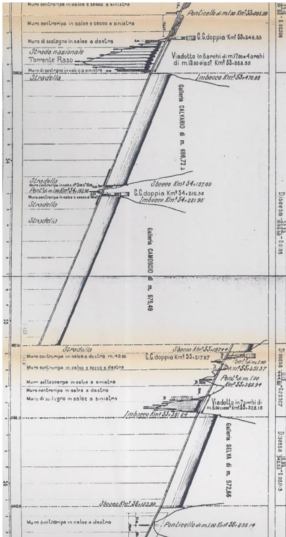
Stralcio del profilo plano-altimetrico della linea ferroviaria
