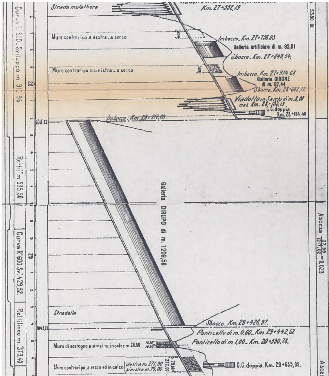
Stralcio del profilo plano-altimetrico della linea ferroviaria
