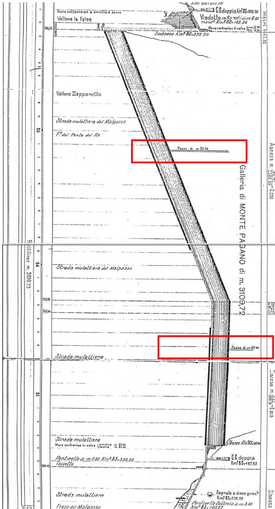
Stralcio del profilo piano-altimetrico della linea
