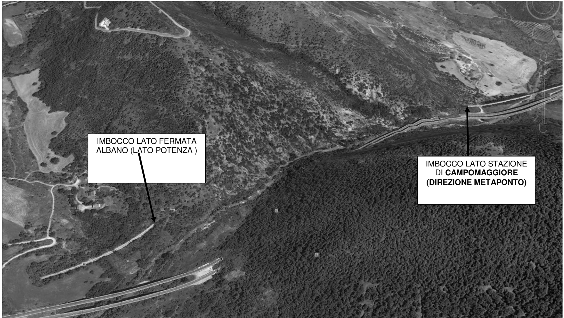
Figura I : ANDAMENTO PLANIMETRICO
