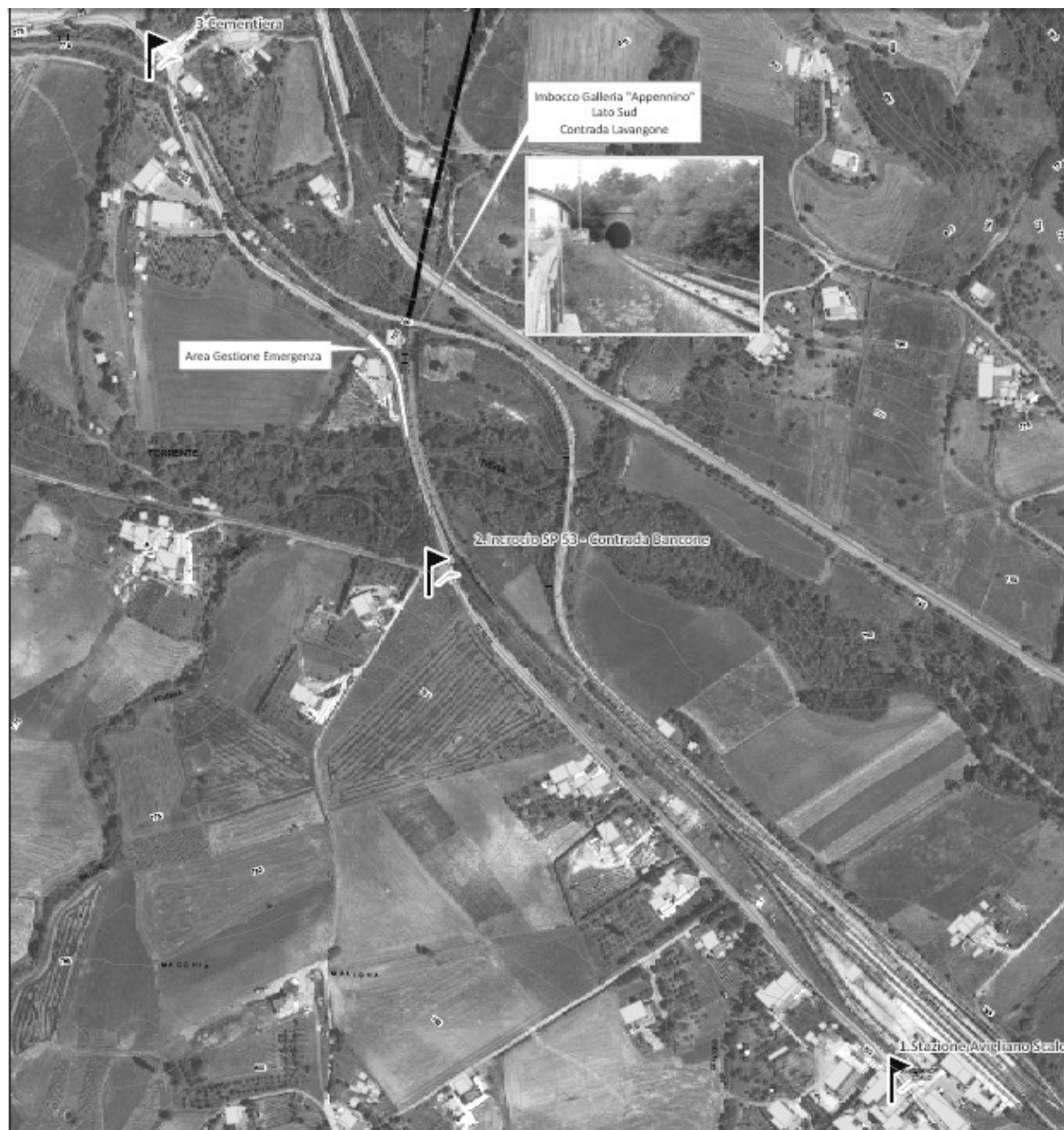
Figura III-7: POSIZIONAMENTO CANCELLI – IMBOCCO LATO AVIGLIANO SCALO (COMUNE DI POTENZA - Contrada Lavangone)
