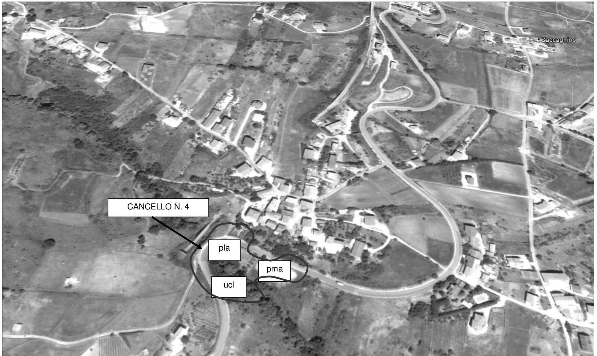
Figura III-6: POSIZIONAMENTO AREE DI INTERVENTO – IMBOCCO LATO STAZIONE PIETRAGALLA SCALO (comune di avigliano)
