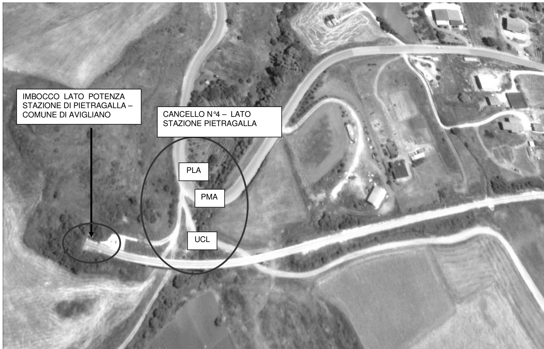
Figura III-4: POSIZIONAMENTO AREE DI INTERVENTO – IMBOCCO LATO SUD - AVIGLIANO (DIREZIONE POTENZA)
