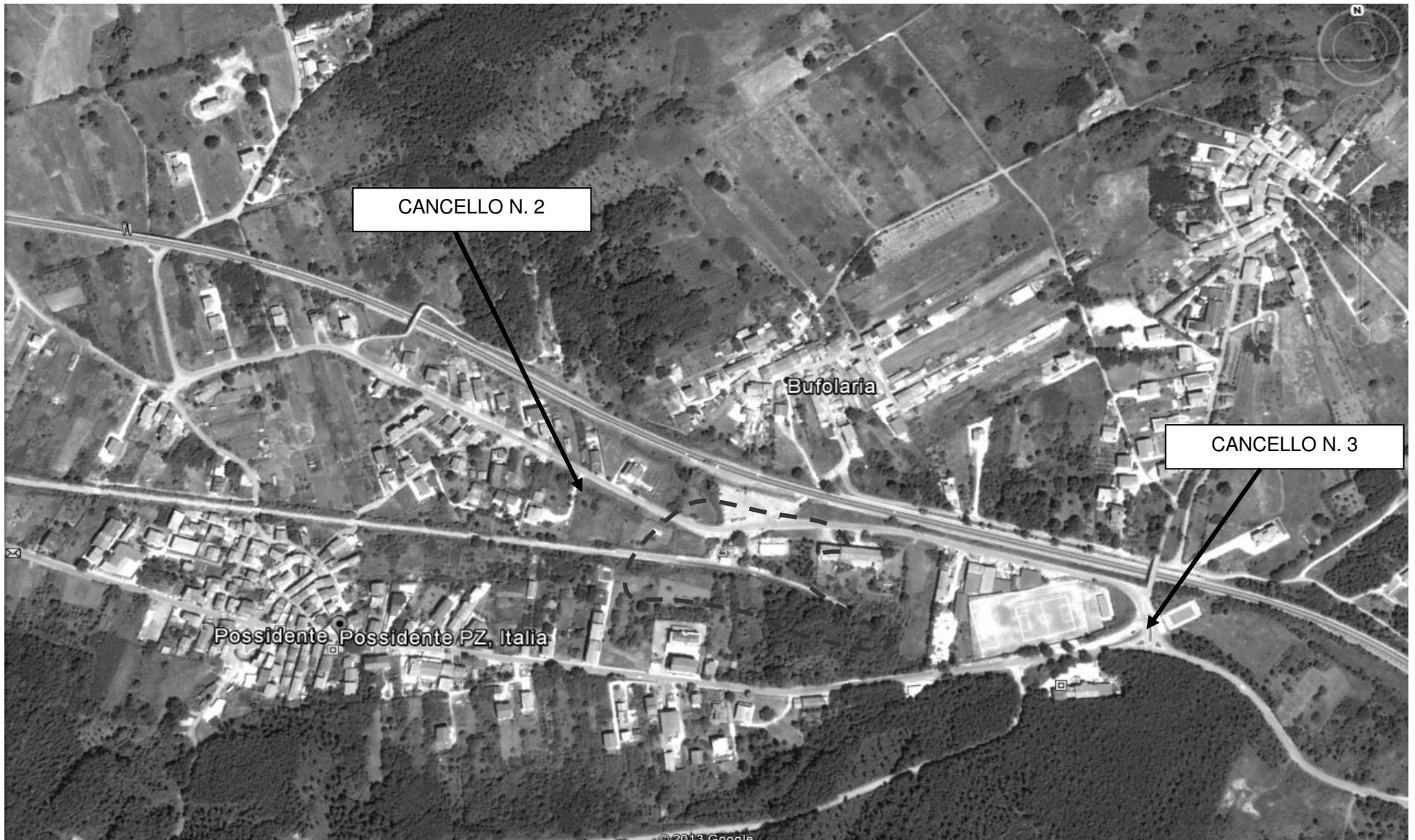
Figura III-5: POSIZIONAMENTO CANCELLI – IMBOCCO LATO POSSIDENTE (DIREZIONE FOGGIA)
